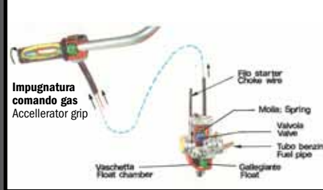
Carburettor
