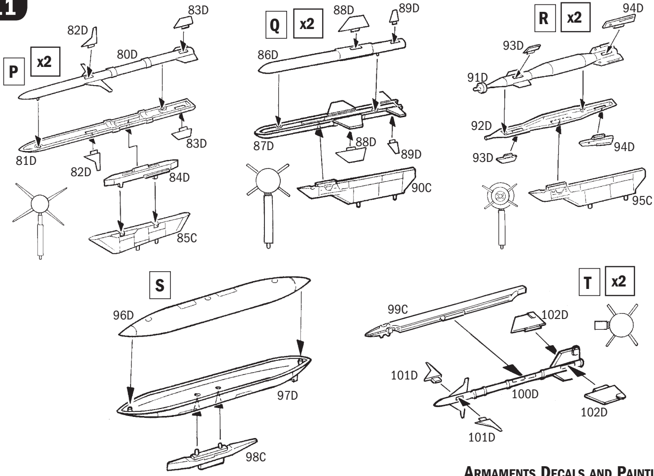
AIM-9L
