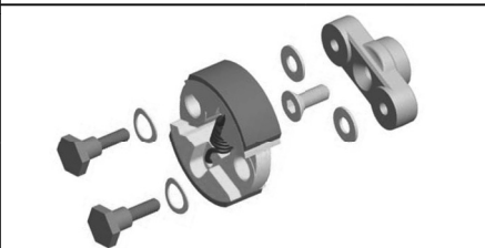
903184 Clutchset Kupplungsset
