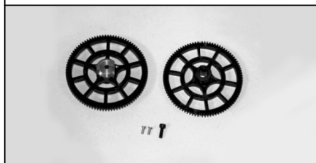
508124 Main gear set Hauptzahnradset BIG EC-135
