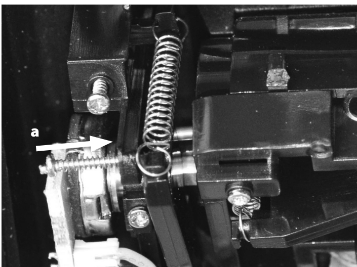
Wichtig: Heben Sie den Hebel an und schrauben Sie Schraube a von der rechten Seite ein.
