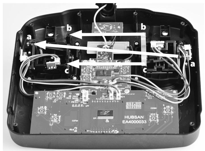
Lösen Sie die Schrauben a, b, c und bewegen Sie die Schrauben b und c und die Feder auf die andere Seite. Schrauben Sie sie an und testen Sie, ob der Hebel sich leichtgängig bewegen lässt.
