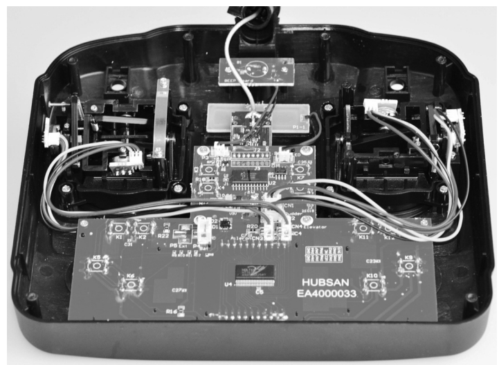
Zum Schluss verschließen Sie die Abdeckung wieder mit den 6 Schrauben. Achten Sie darauf, dass keine Kabel gequetscht werden.
