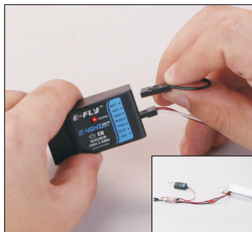
2. 给接收机供电, 接收机显示灯开始闪烁, 在BATT处插上短路插(如图所示).
