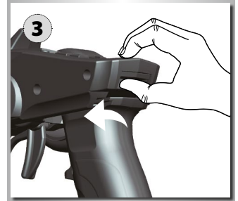
3 Handgriff installieren
