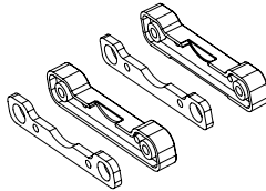
500405970 Querlenkerhalter unten hinten / Lower suspension mount rear
