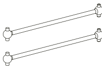
500405910 Antriebswellen Mitte (2) Center drive shaft (2)
