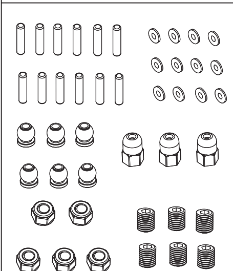
50 040 5340 24x Unterlegscheiben, 12x Pin, 6x Kugelkopf-, 18x Schrauben, 5x Klemmmutter 24x Washer, 12x pin, 6x d. way ball end, 18x screw, 5x locknut
