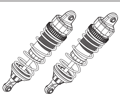
50 040 5312 2x Stoßdämpfer (Kunststoff) 2x Shock absorber unit (plastic)
