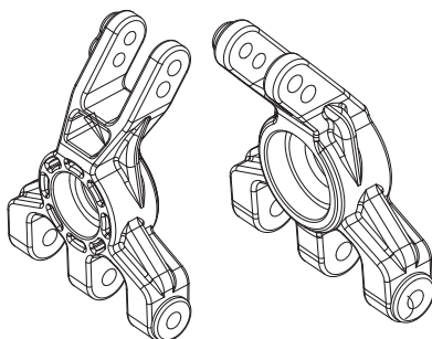
50 40 5273 Nabenhaltung hinten Hub rear carrier
