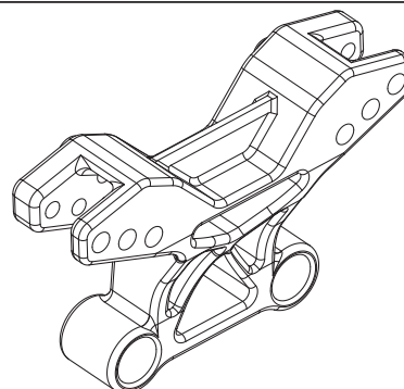
50 040 5289 Dämpferbrücke Shocktower
