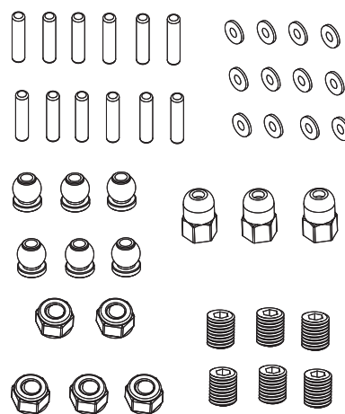
50 040 5340 24x Unterlegscheiben, 12x Pin, 6x Kugelkopf-, 18x Schrauben, 5x Klemmmutter 24x Washer, 12x pin, 6x d. way ball end, 18x screw, 5x locknut
