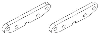
50 040 5258 Querlenkerhalterung oben v + h Upper suspension mount f + r
