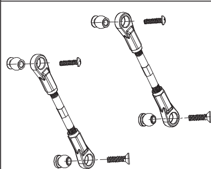
50 040 5324 2x Lenkgestänge 2x Steering linkage
