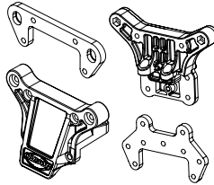
500405982 Shock towers front/rear (2) Dämpferbrücken v/h (2)
