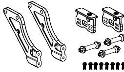
500405980 Alu Shocks-kit v/h Alu Stoßdämpfer-Set v/h
