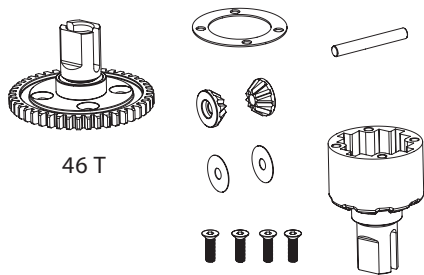
500405592 Centerdiff complete Mitteldiff komplett
