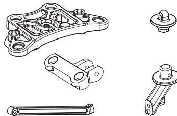
500405621 Bodyholder-Kit Karosseriehalter-Set
