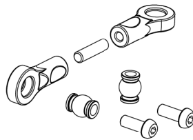
500405213 Servo link Servogestänge
