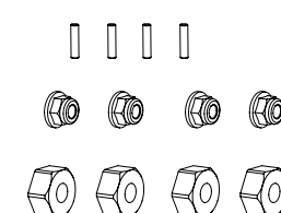
500405799 Felgenmitnehmer 12mm Kant (4) / Rim hub 12 mm
