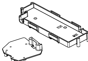
500405782 Akkuhalterung Battery holder
