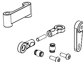
500405798 Lenkgestänge-Set vorne suspensions holder
