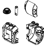
8 Gearbox cover Getriebegehäuse
