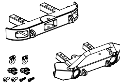
20 Bumper front/rear Stoßfänger vorne/hinten
