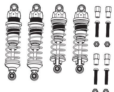
500405414 4x Stoßdämpfer-Set v/h 4x Front/rear shock set
