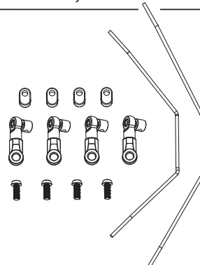
50 040 5416 Stabilisator Set vorne/hinten Sway bar set front/rear
