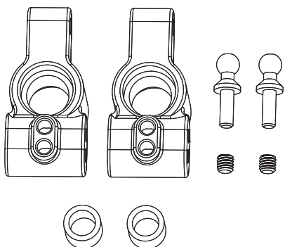
50 040 5354 2x Achsschenkel-Set hinten 2x Rear hub set
