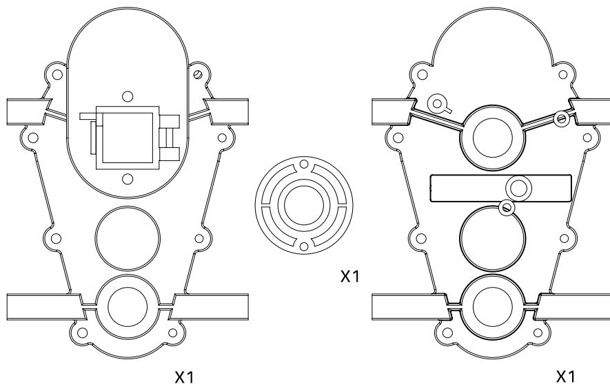
205061 Two Speed Gear Box / Gehäuse 2-Gang-Getriebe
