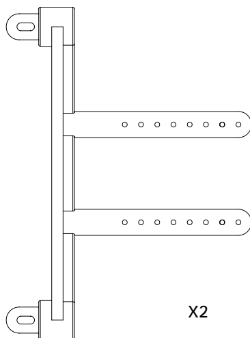
205122 Body Holder / Karosseriehalter
