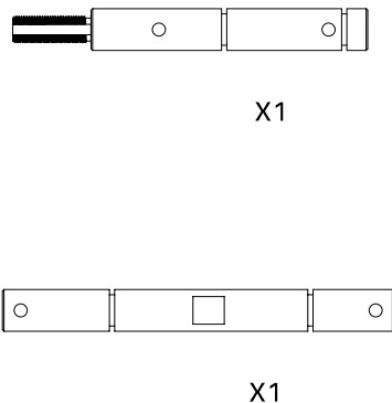
205068 First Gear Holder / Halterung 1. Gang
