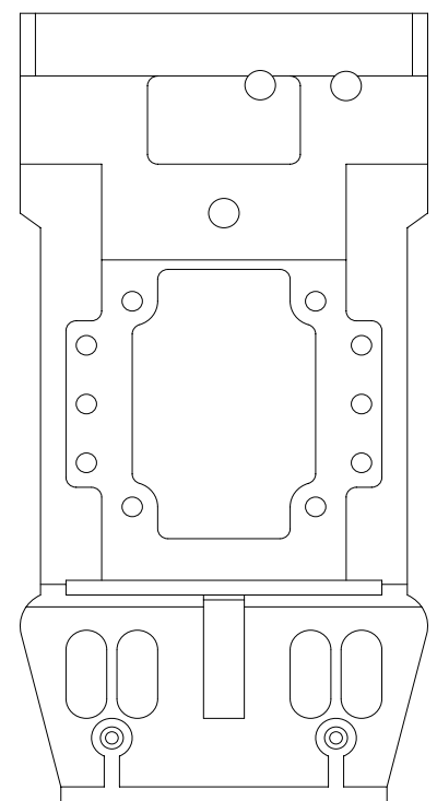
205058 Skid Plate / Unterbodenschutz
