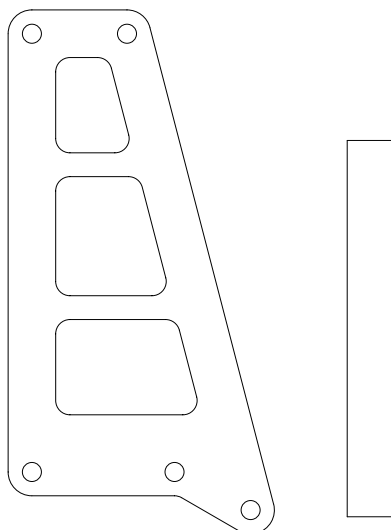
205074 Handle Bar / Überrollbügel
