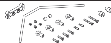
205349 Suspensionholder front alu 0° Unterer Querlenkerhalter 0° Alu vorn
