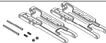
205326 Hub carrier l-r blue Lenkhebelaufnahme l-r Alu blau
