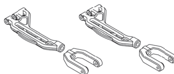
205292 Upper suspension plate f+r Querlenkergegenhalterung f+h
