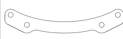
500205788 2x Engine mounts 2x Motorblöcke Alu
