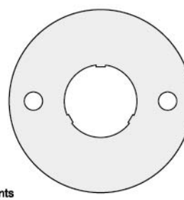
MA14 ×1 モータープレート Motor plate Motor-Platte Plaque-moteur
