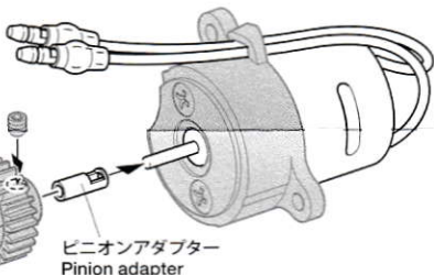
370トルクチューンモーター Type 370 Torque-tuned motor
