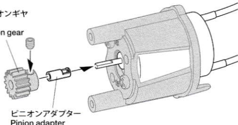
ピニオンアダプター Pinion adapter
