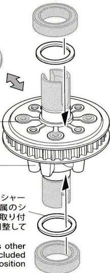
ギヤデフプーリーケース Differential case
