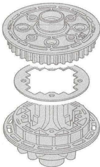
37Tギヤデフプーリー Differential pulley
