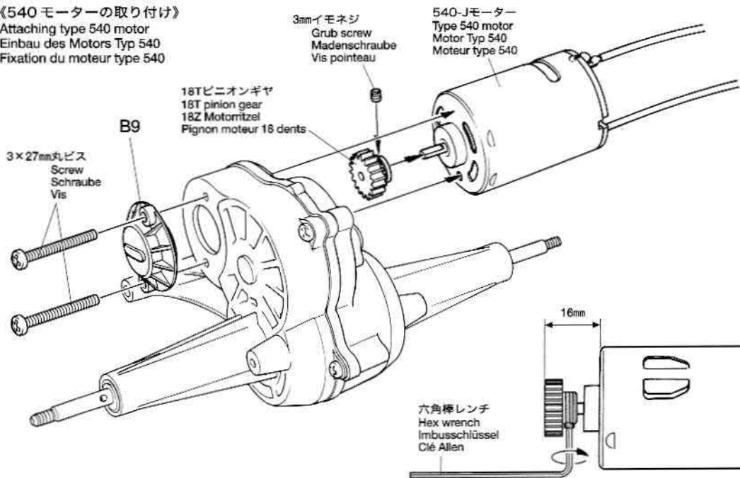
18Tピニオンギヤ 18T pinion gear 18Z Motorritzel Pignon moteur 18 dents
