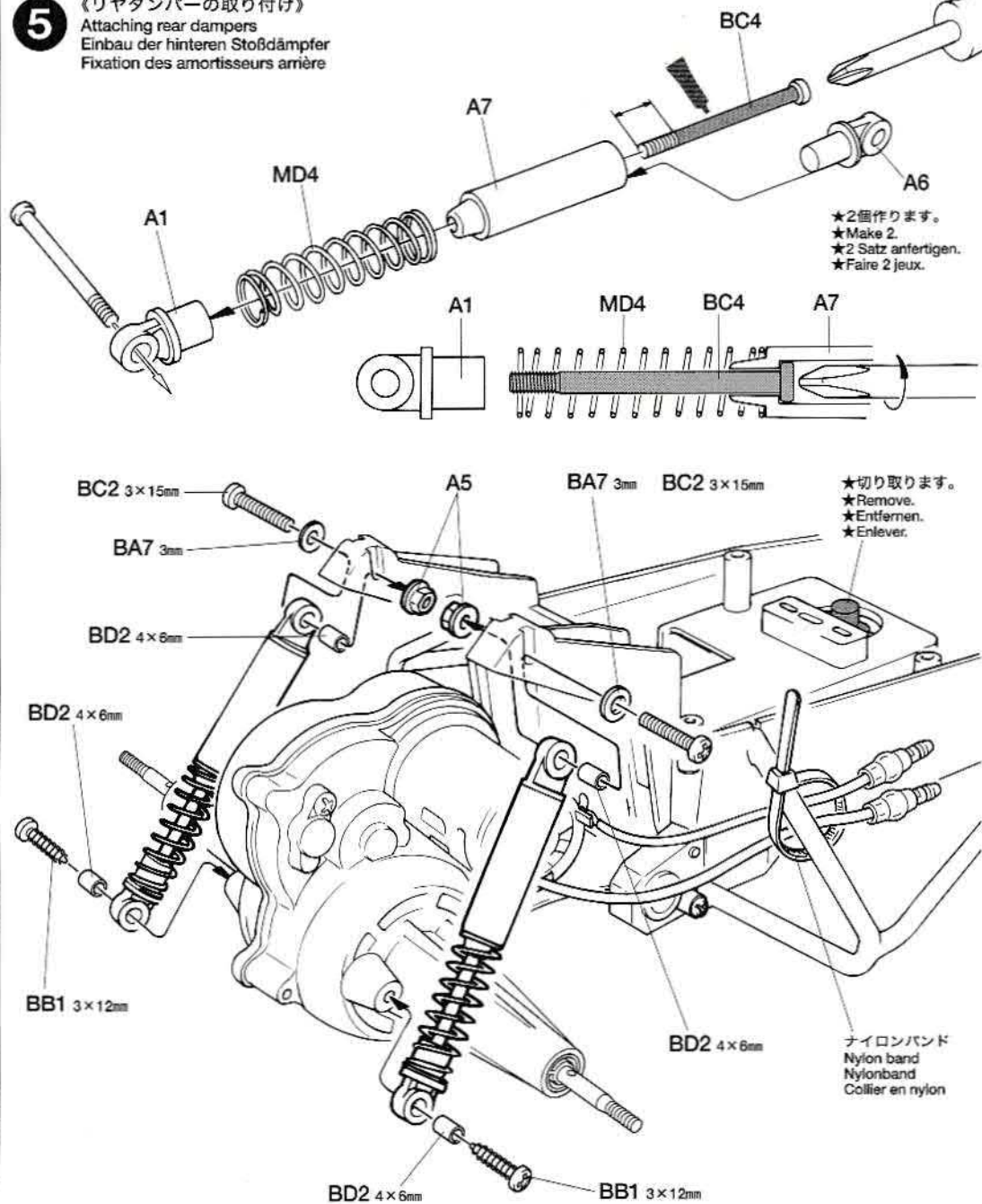
MD4 × 2 リヤコイルスプリング Rear coil spring Hintere Spiralfeder Ressort hélicoïdal arrière
